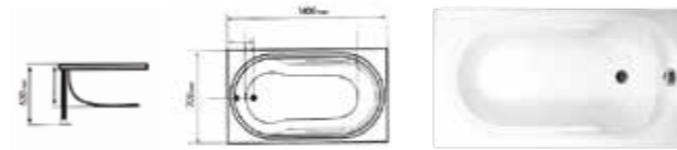
MODEL MITRA (میترا) Size: 1500 * 700 * 570mm
