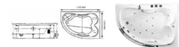
MODEL DIYANA (دیانا) Size: 1700 * 1200 * 560mm
